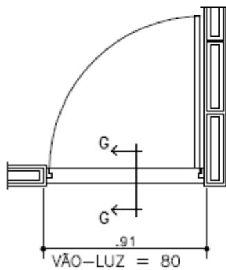
P3 PORTAS INTERNAS PLANTA ESC. 1:25
