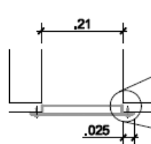
PLANTA ESC. 1:10
