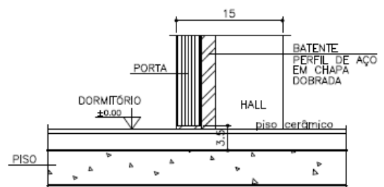
CORTE C-C ESC. 1:5
