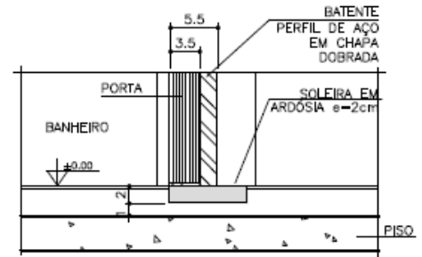
CORTE A-A ESC. 1:5
