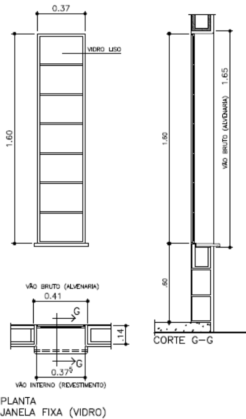
VISTA EXTERNA ESC. 1:10
