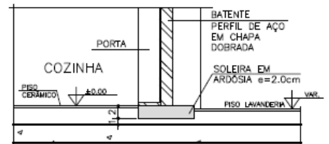
CORTE B-B (COZINHA) ESC. 1:5
