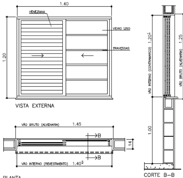
PLANTA JANELA DE CORRER(VENEZIANA) 3 folhas { 1 veneziana de correr 1 veneziana de correr (c/ ventilação) 1 vidro de correr com travessas
