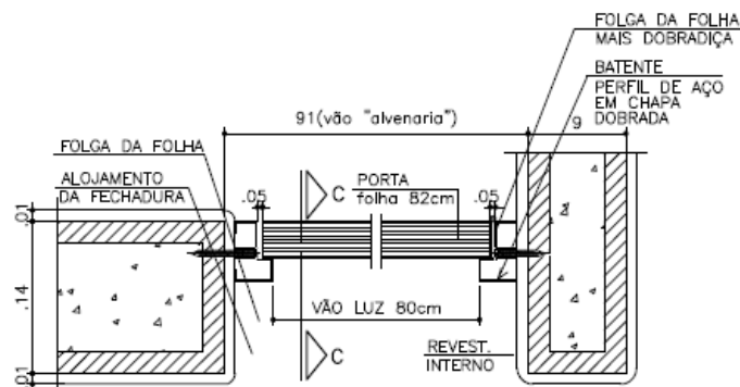
DET. PORTA-DORMITÓRIO ESC. 1:5
