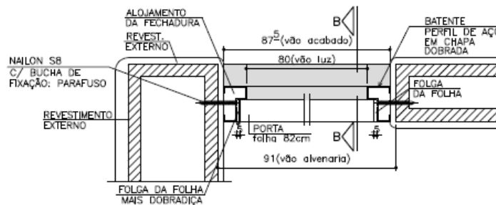
DET. PORTA-COZINHA (EXTERNA) ESC. 1:5
