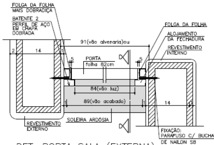
DET. PORTA SALA (EXTERNA) ESC. 1:5
