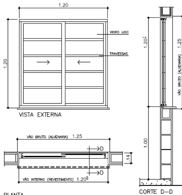
PLANTA JANELA DE CORRER(VIDRO) 2 folhas { 2 vidros de correr c/ travessas
