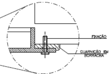
DETALHE ESC. 1:2
