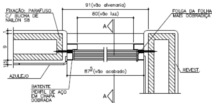
DET. PORTA-BANHEIRO ESC. 1:5
