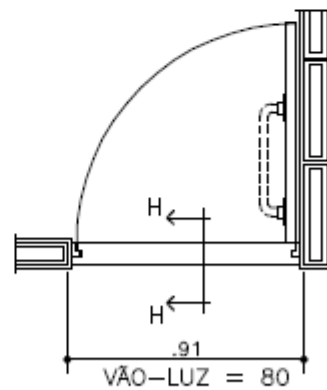
P4 PORTAS INTERNAS P/ UNIDADES ADAPTADAS PLANTA ESC. 1:25 PREVER BARRA NA PORTA DO BANHEIRO VER F. 07/08
