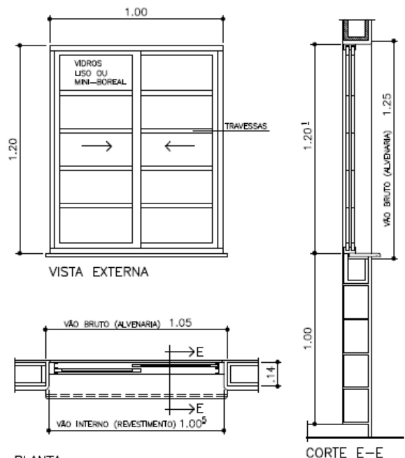
PLANTA JANELA DE CORRER(VIDRO) 2 folhas { 2 vidros(mini-boreal ou liso) de correr.
